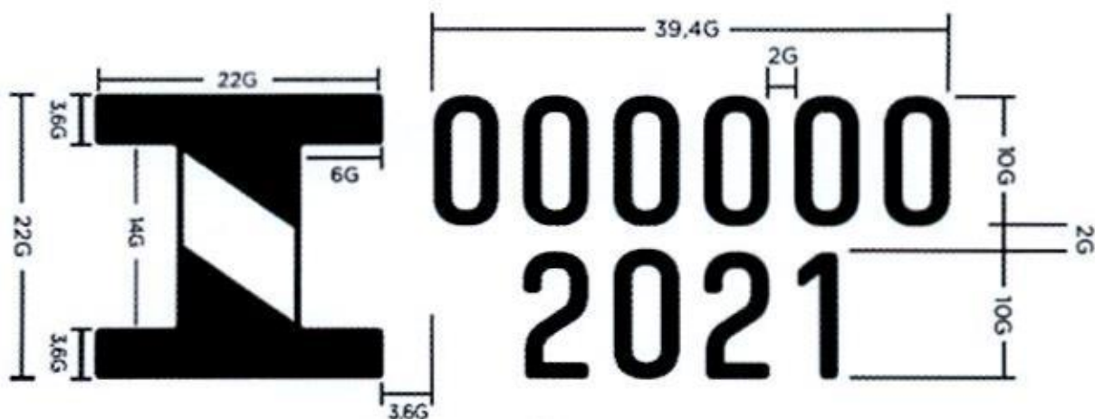
Molde (G mínimo = 0,25mm)
