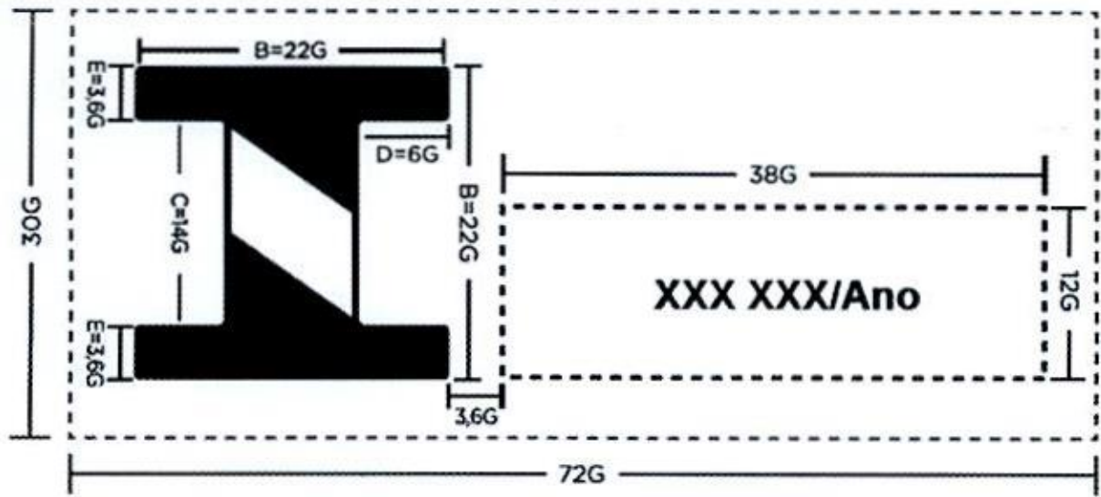
Molde (G mínimo = 0,25mm)
